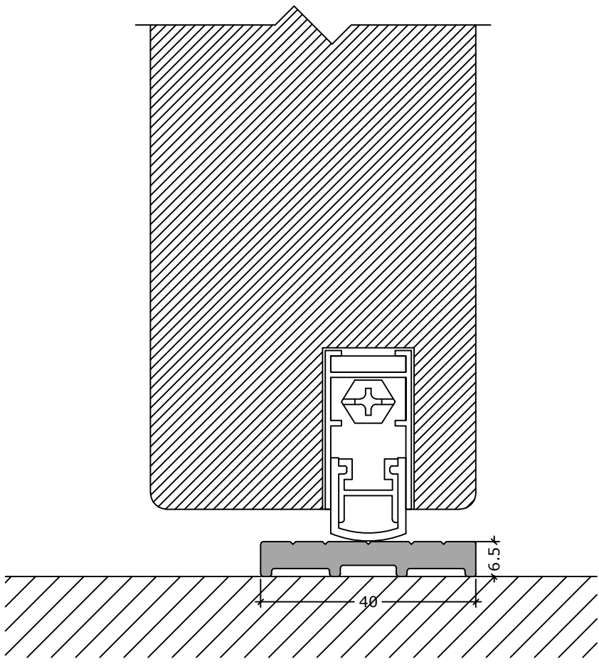
DEKO TD 62mm solid door
