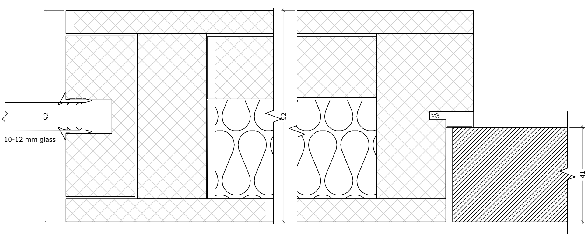
DEKO PD detail (Portal door)
