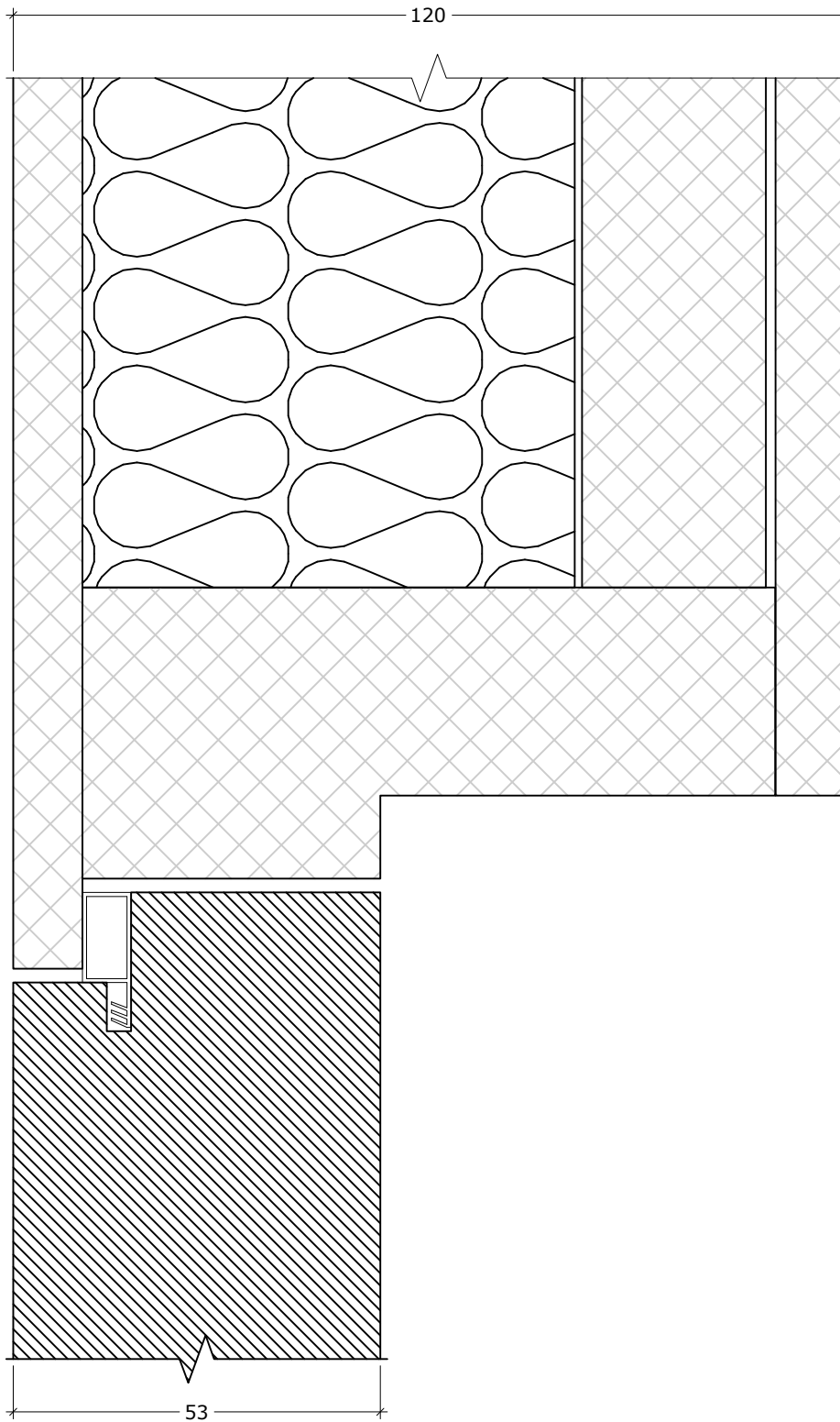
DEKO PD detail (Portal door)
