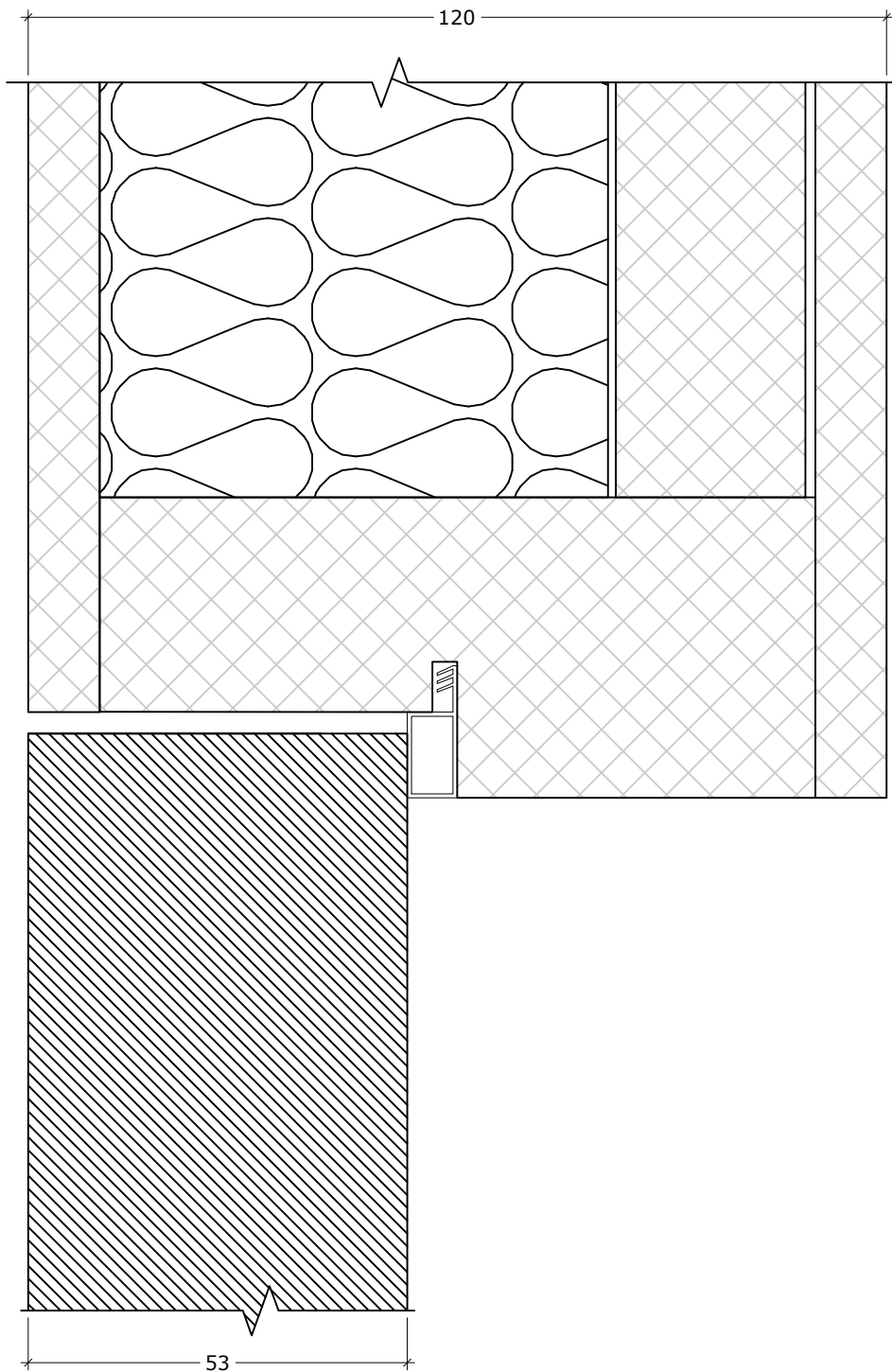
DEKO PD detail (Portal door)
