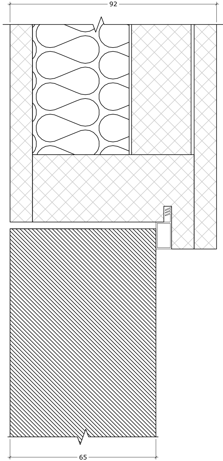
DEKO PD detail (Portal door)
