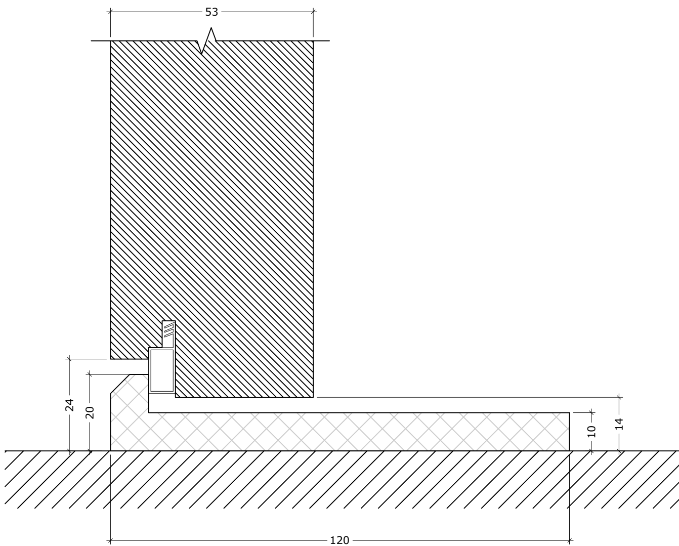
DEKO PD detail (Portal door)
