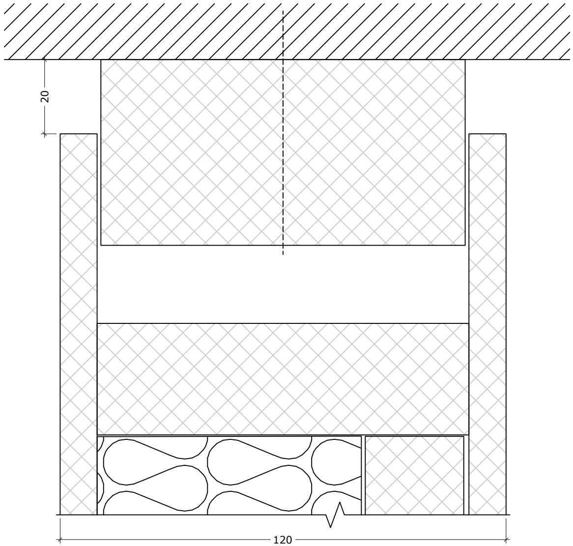
DEKO PD detail (Portal door)
