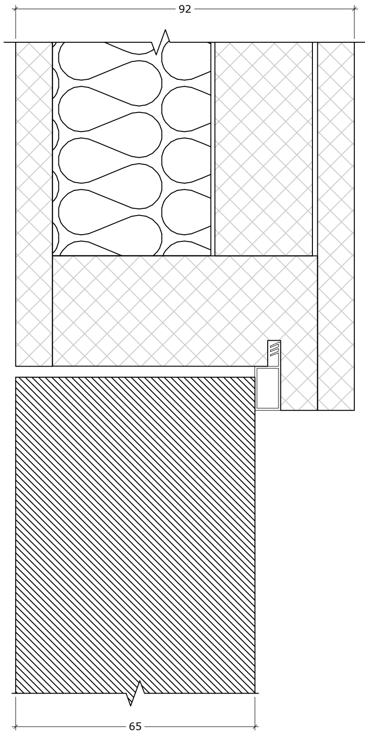
DEKO PD detail (Portal door)
