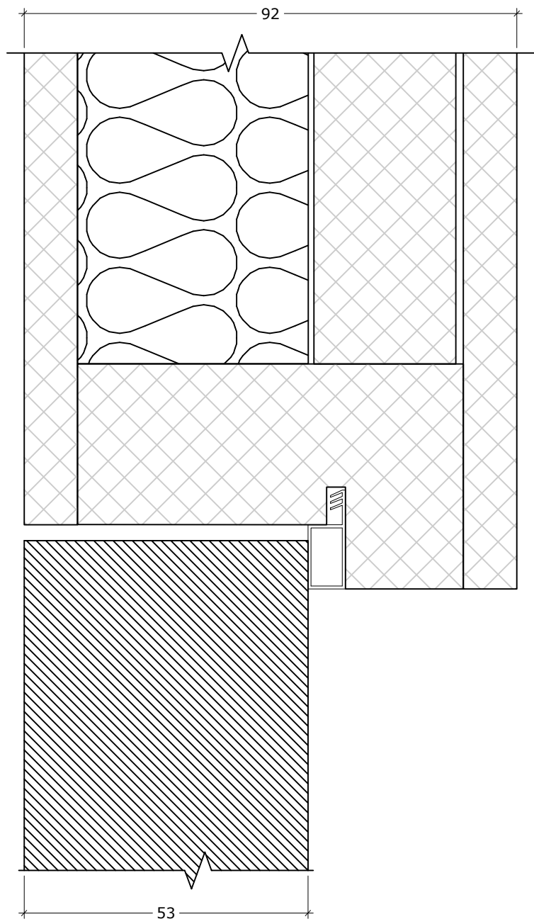
DEKO PD detail (Portal door)
