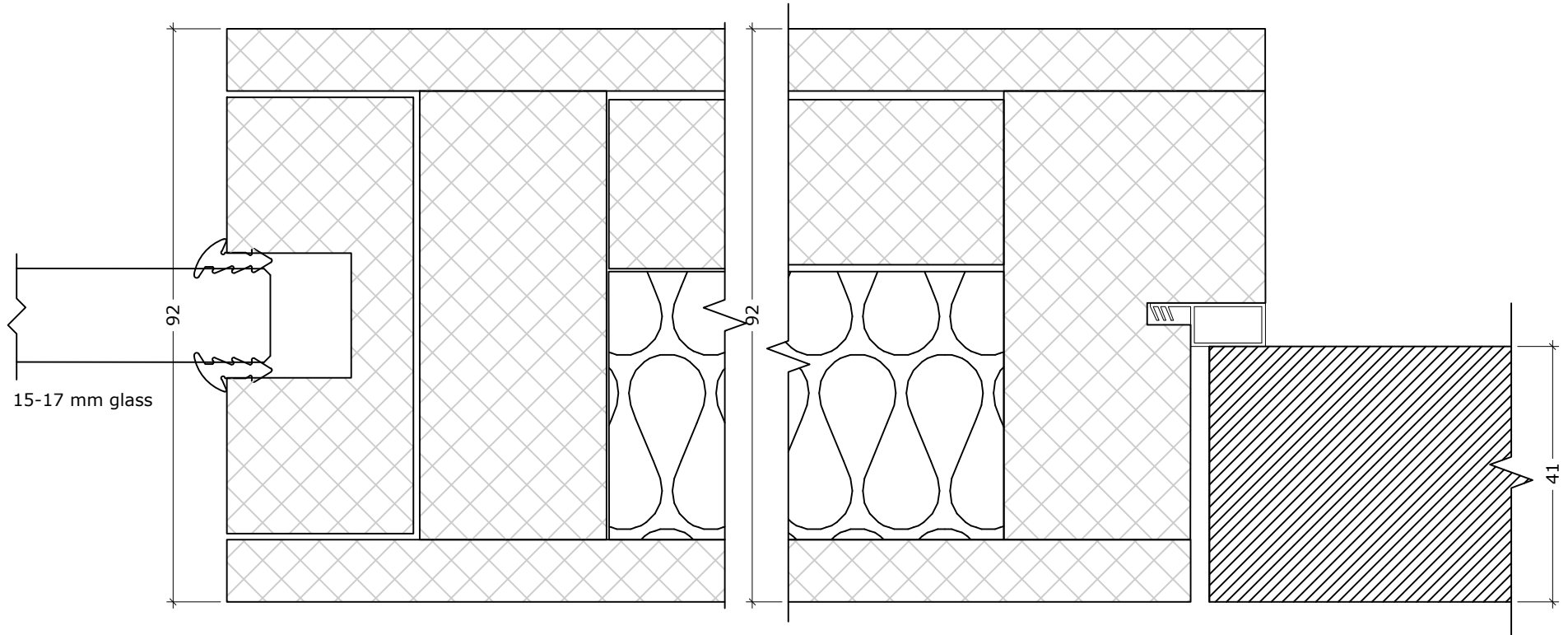
DEKO PD detail (Portal door)
